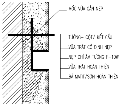
MẶT CẮT
